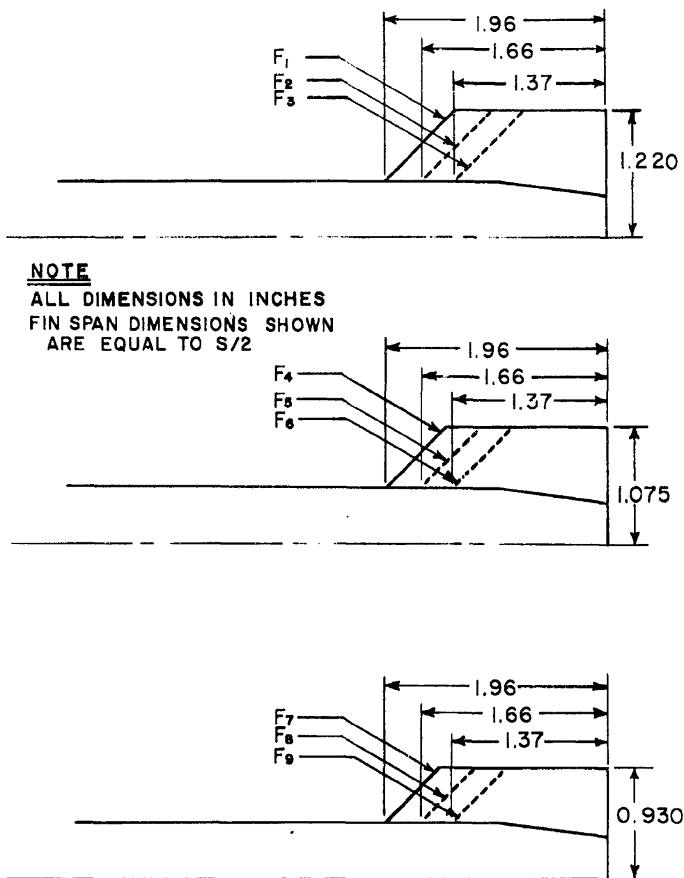
FIG. 2 HOPI WEAPON FIN DIMENSIONS
