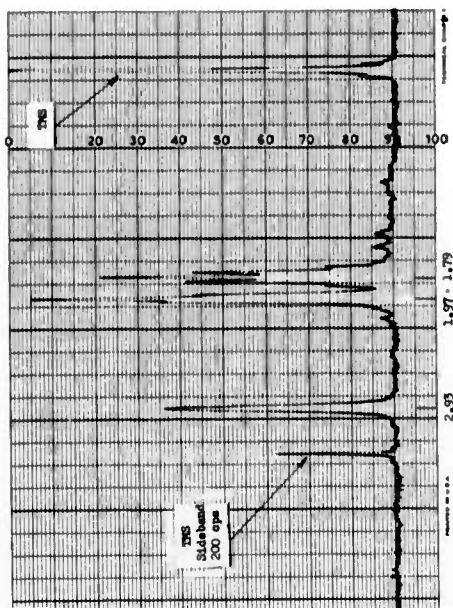
Fig. 18 Proton NMR Spectrum of 2-Chloro-2,4,4-tris(difluoramino)pentane
