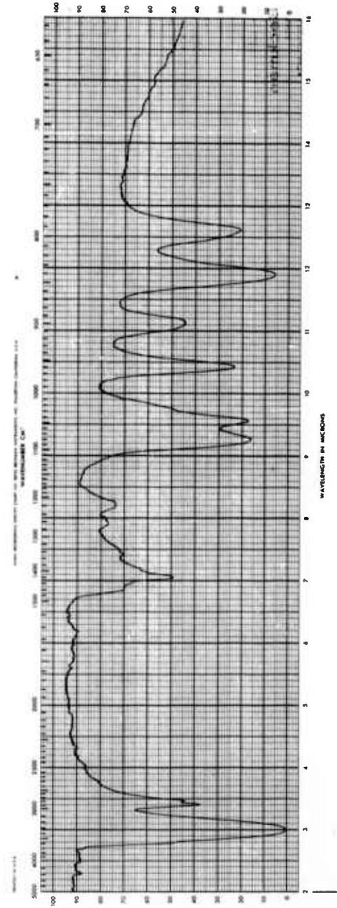
Fig. 30 Infrared Spectrum of \beta -Difluoroaminoethanol
