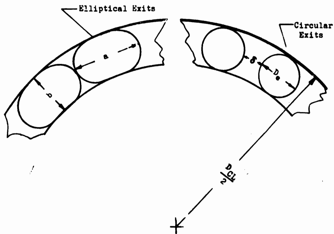
Fig. 114 Multichamber Nomenclature
