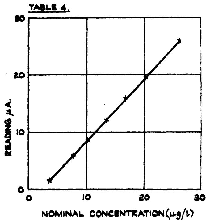
(d) HEXANE.
