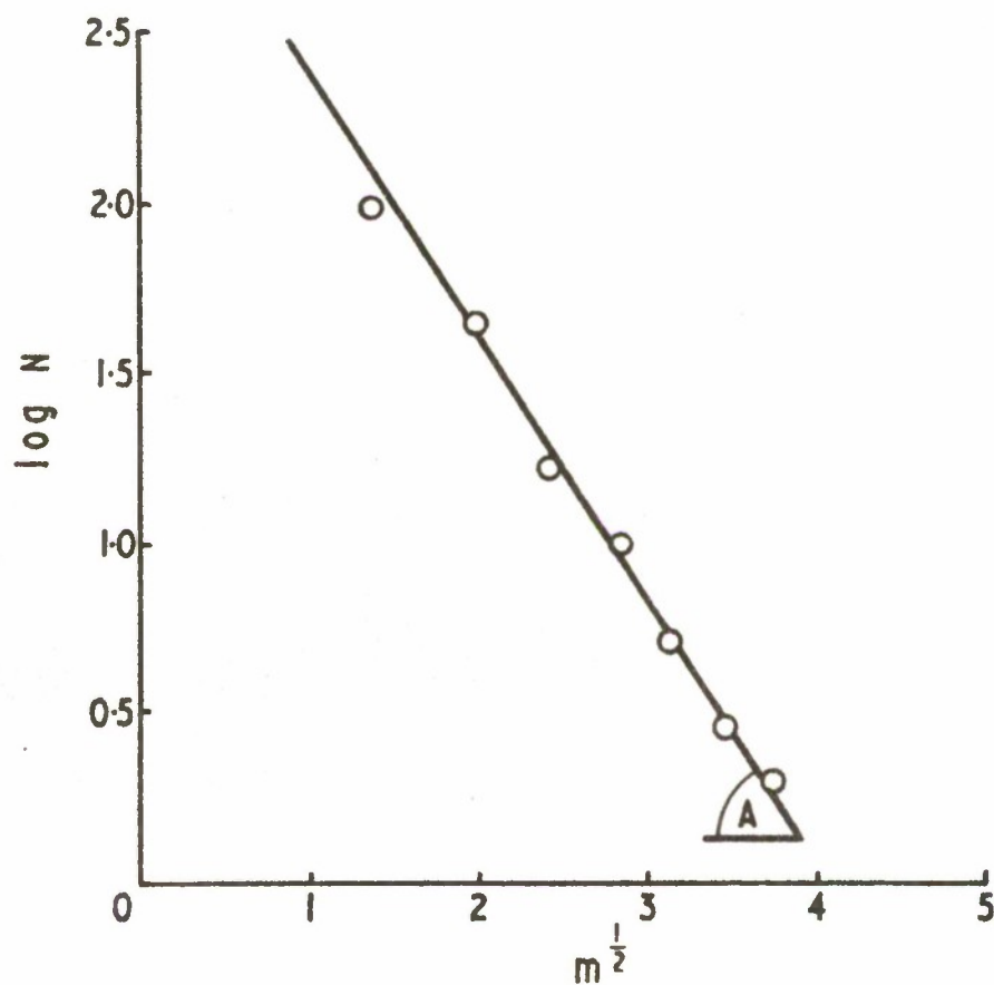
FIG. I NUMBER - MASS PARAMETER \hat{A} (100 g RDX CHARGE)
