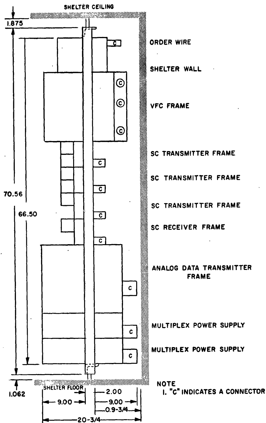
Figure 3-10. PAR Microwave Terminal, Profile Rack No. 2
