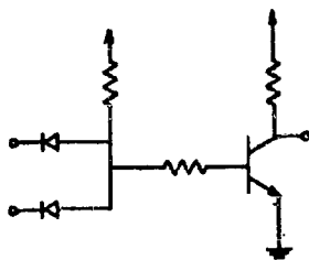
DTL-NOR
