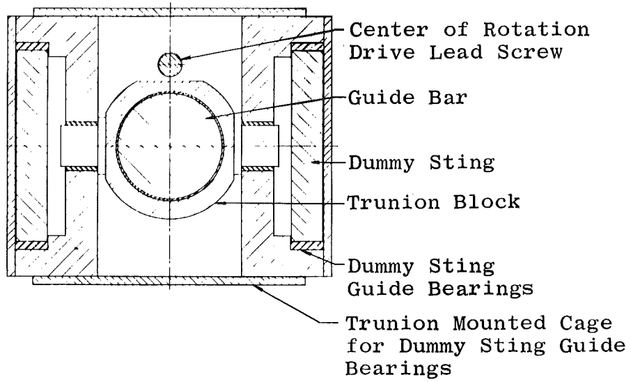
Section D-D
