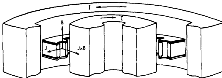
Fig. VIII-8. Homopolar device.
