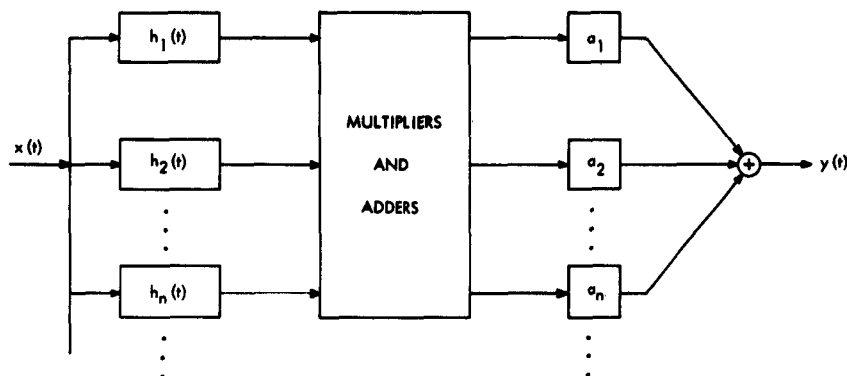
Fig. IX-9. Nonlinear system.
