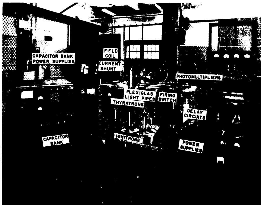
Fig. VIII-9. Rotating-plasma apparatus.
