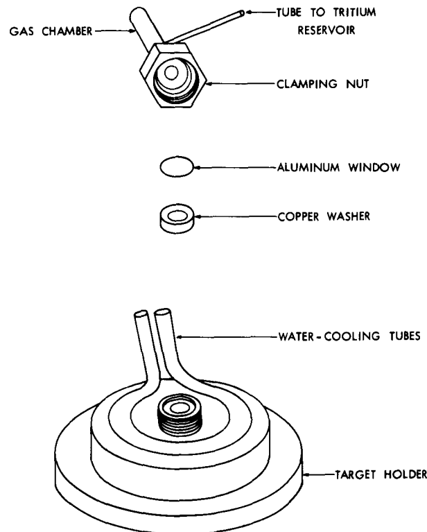
Fig. VII-25. Gas target.
