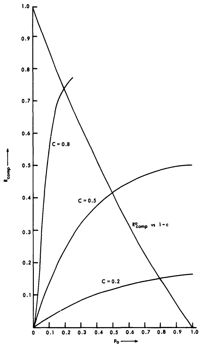
Fig. X-7. R_{comp} versus p_o .
