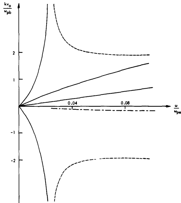
Fig. VII-17. Longitudinal dispersion n_b/n_p = 10^{-2} , T_e/2V_0 = 25 .
