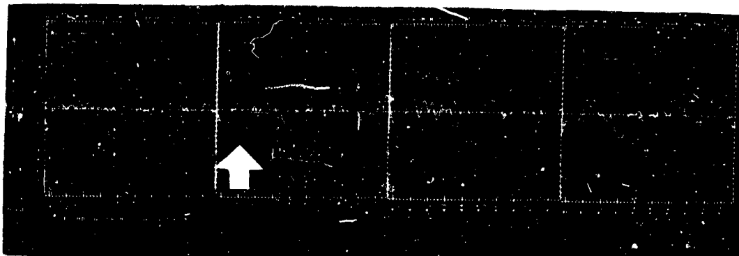
Original Seismogram
