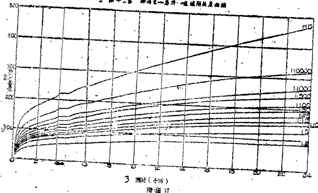
1 第十二區 降雨量—雨時—雨量關係曲線
