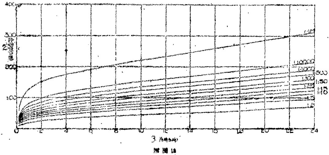
圖 13 第十三區 降雨量—小時—頻率關係曲線
