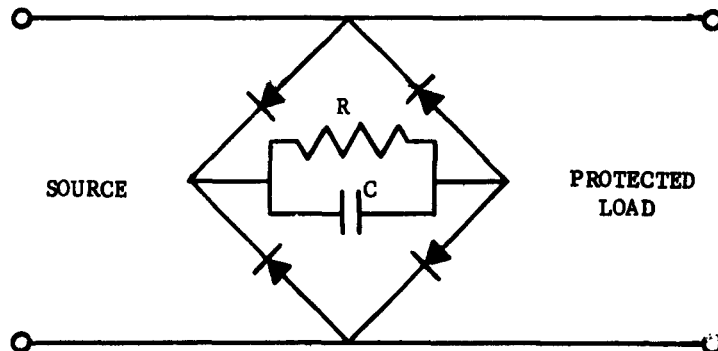
(d) Diode Bridge R-C Suppressor
