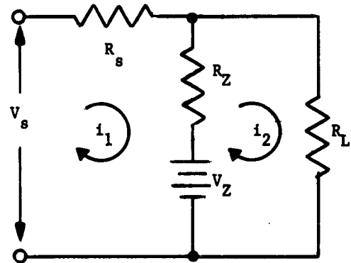
(d) Equivalent of Protective Circuit for V_s Above Diode Breakdown Voltage
