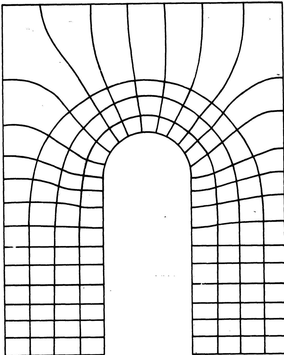
Fig. 4-7. Equipotential and Equipotential Lines for Rounded Corner
