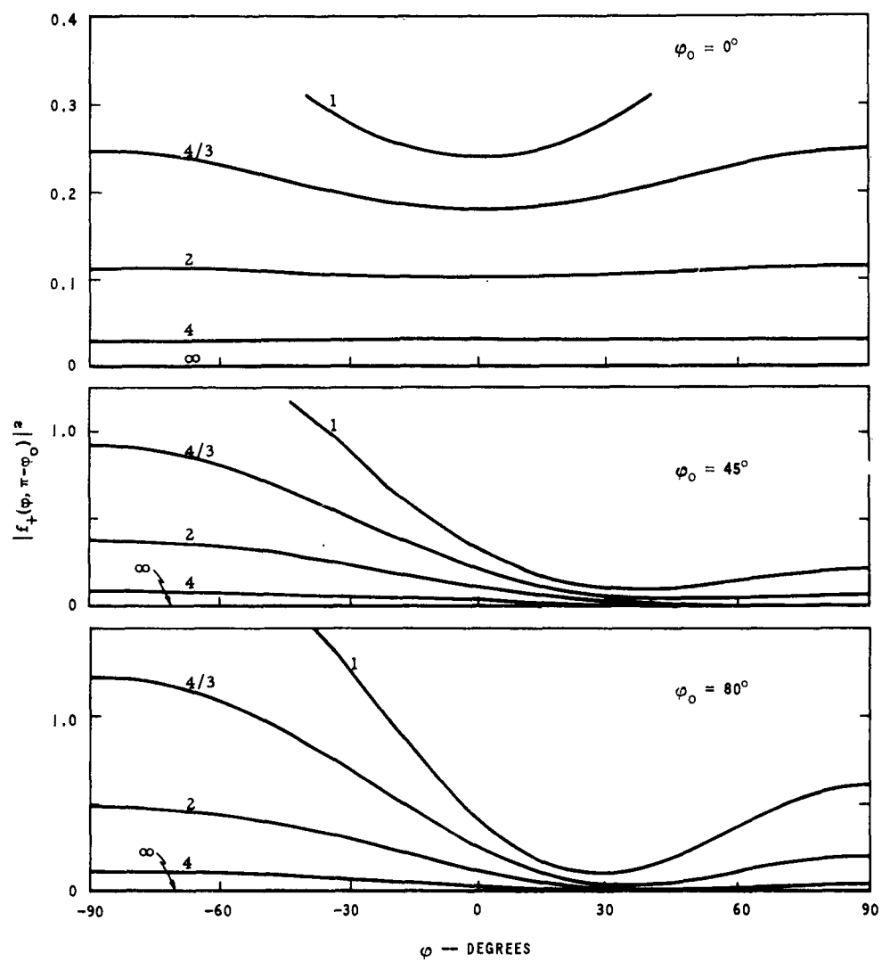
Graph III-7 (con't): ka = 0.7
