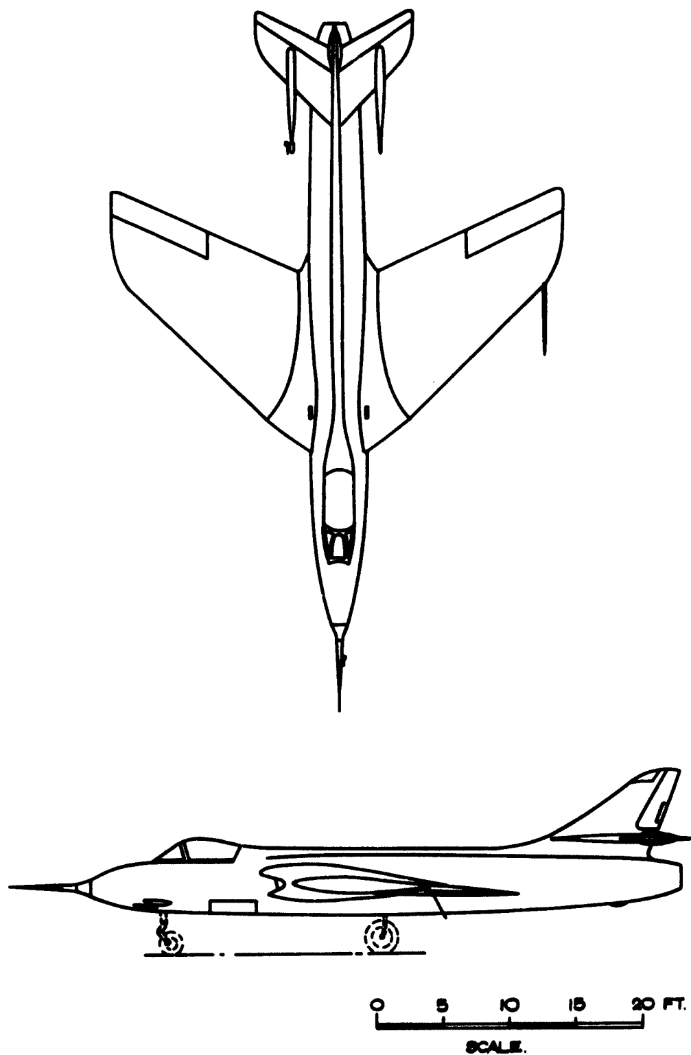
FIG. 2. HAWKER HUNTER F.2. (WN.893.)
