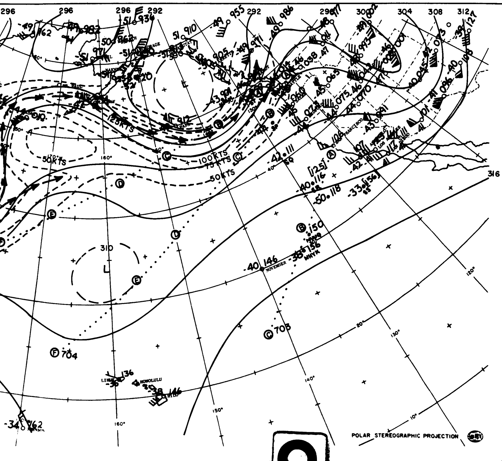
FIG. 11 300-mb MAP, 20 MAY 1960, 0000 G.M.T.
