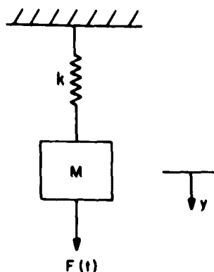
Fig. 1 - Linear oscillator
