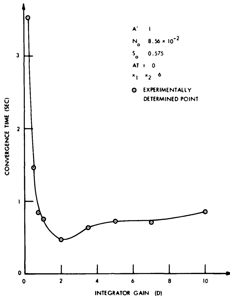
Fig. XIV-14. Convergence time versus integrator gain (D).
