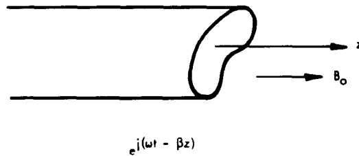
Fig. XII-17. Beam-plasma system.
