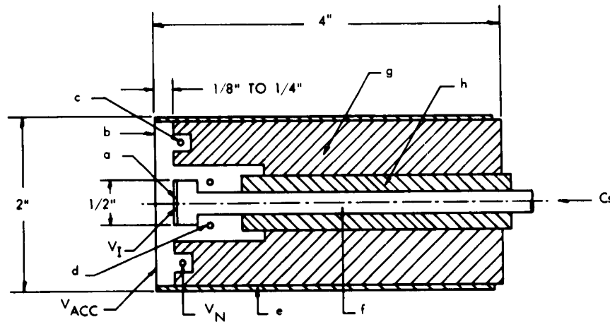
Fig. XII-36. Cesium ion source.
