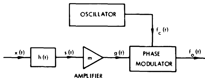
Fig. XIV-18. Phase-modulation system.
