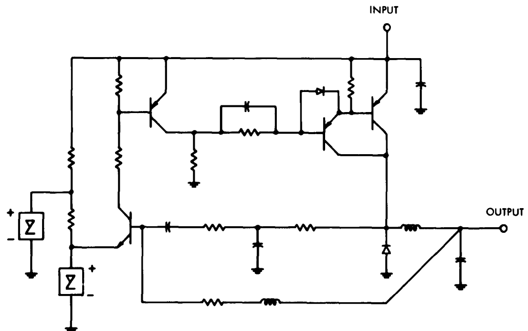
Fig. XIV-8. A dc transformer.
