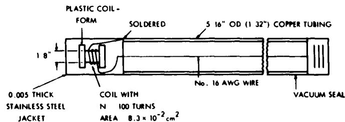
Fig. XII-1. Magnetic probe.
