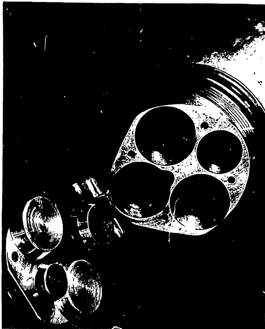
FIG. 31. Nozzle Plate.
