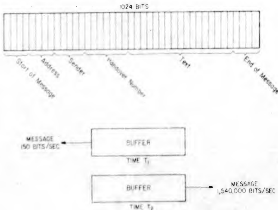
FIG 10 -- Message Block
