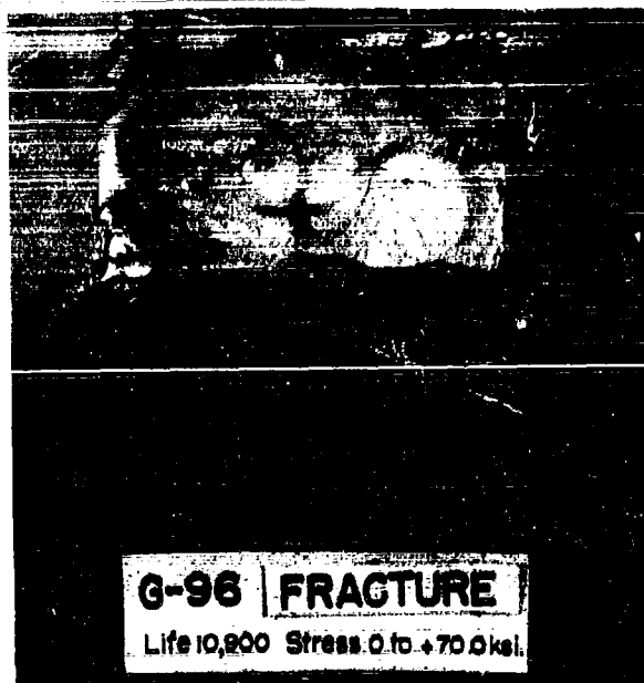
b) SLAG IN WELD.
