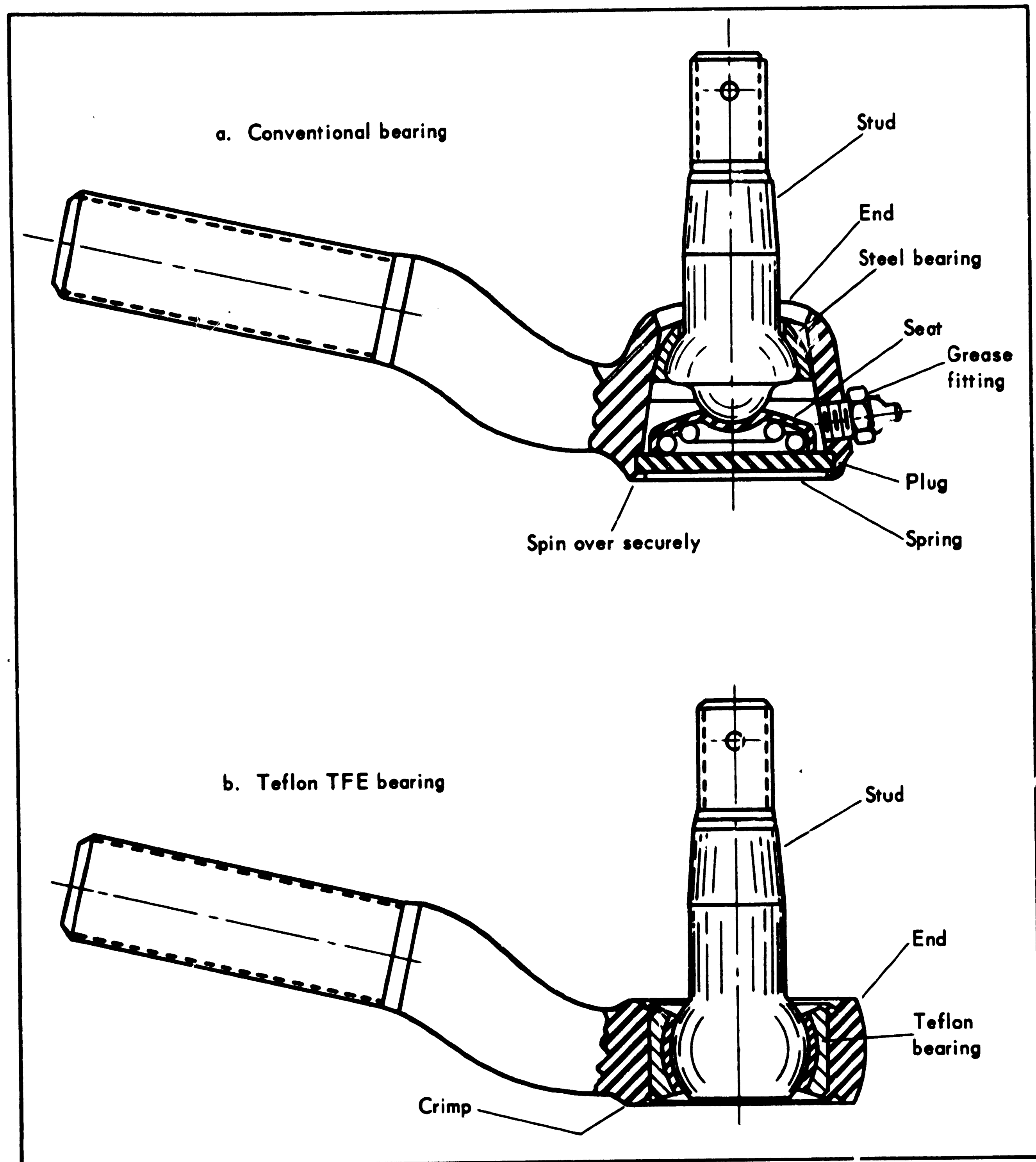
Fig. 10—Rod End
