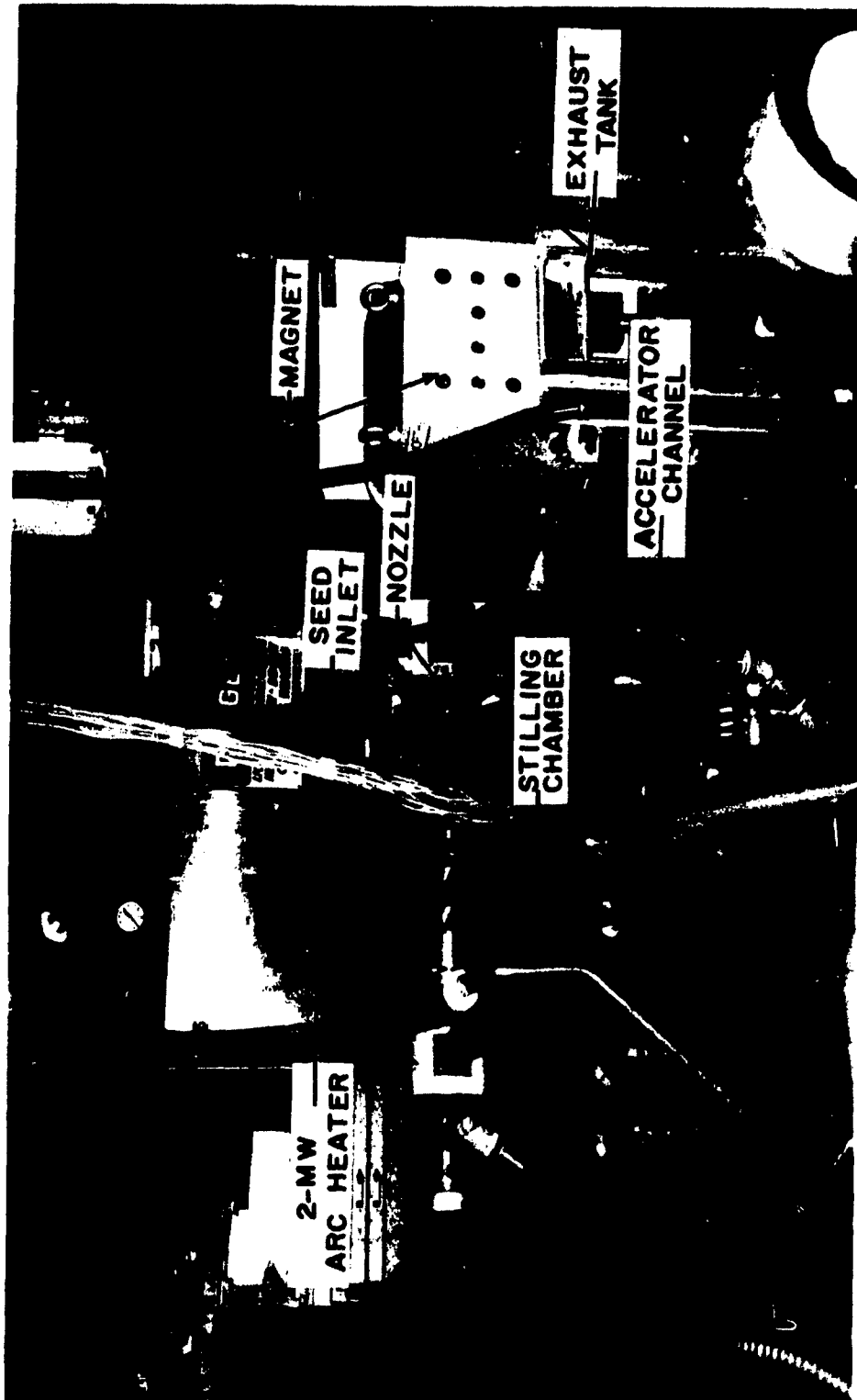
Fig. 4 Test Apparatus
