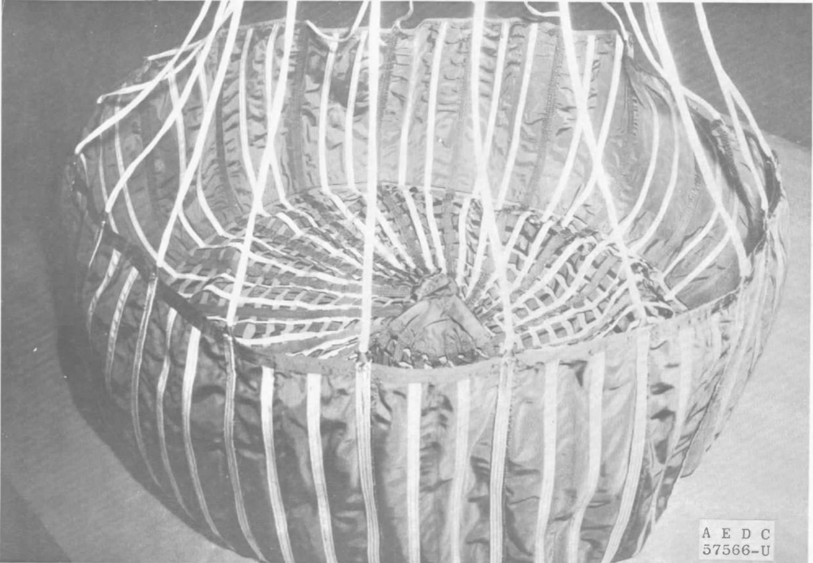
Fig. 13 Hemisflo Parachute
