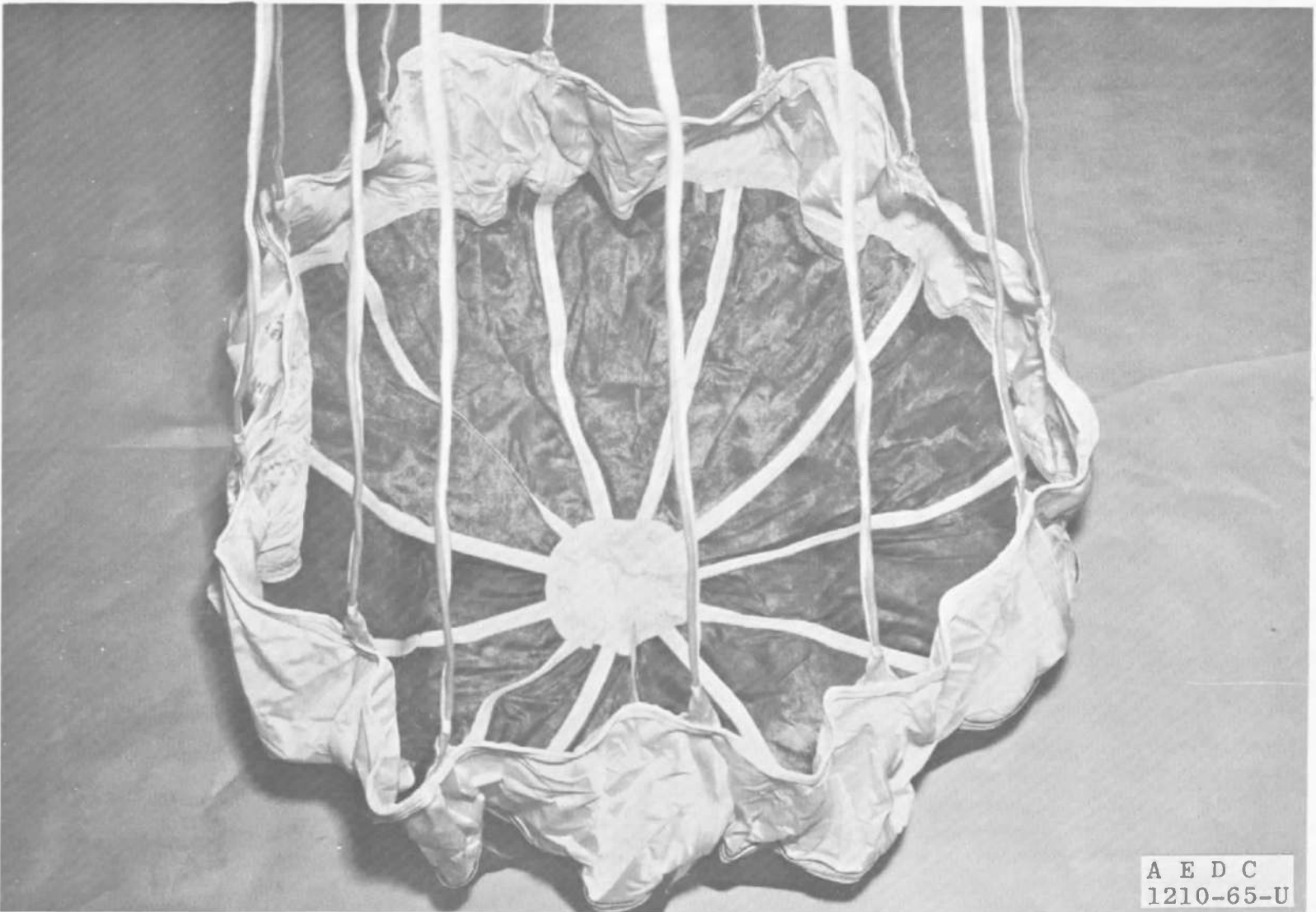
Fig. 11 Parasonic Parachute
