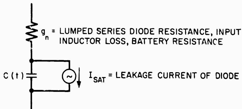
Fig. C-1. Diode model.
