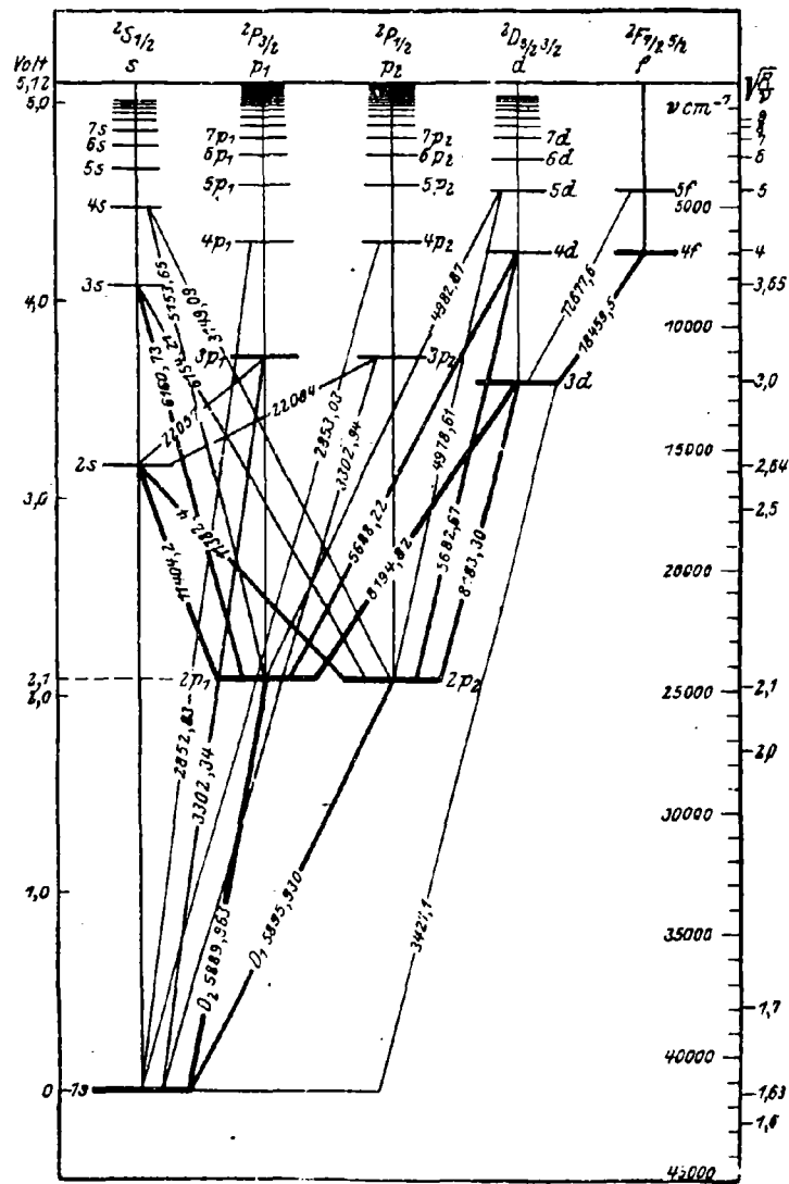
Fig. 18, II, Text S. 63 Niveauschema des Natrium I.
