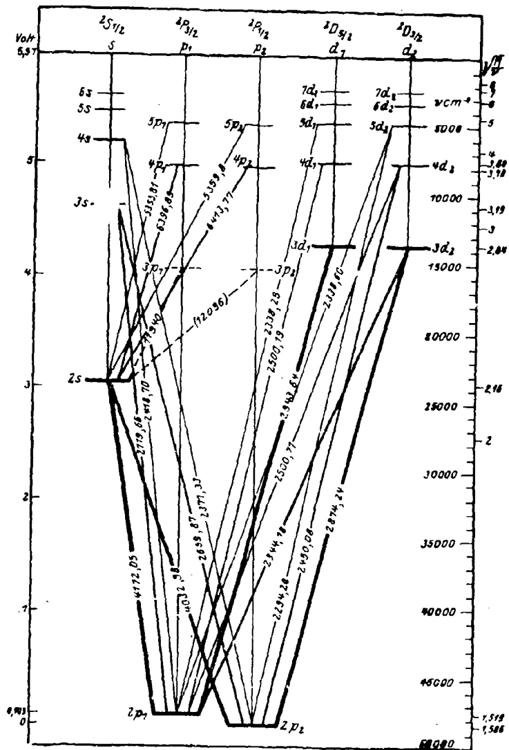
Fig. 89, II, Text S. 123. Niveauechema des Gallium I.
