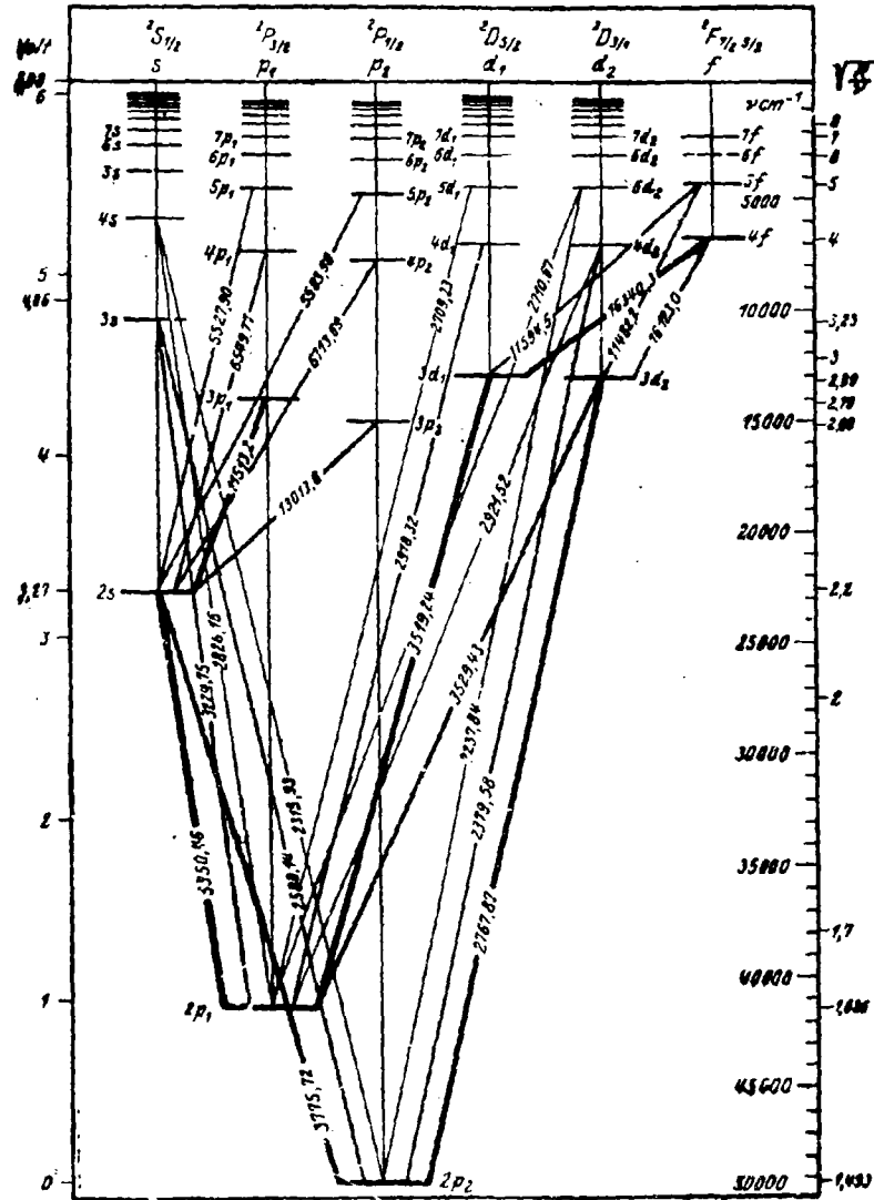
Fig. 95, 11, Text 9. 128. Niveauschema des Thallium I.
