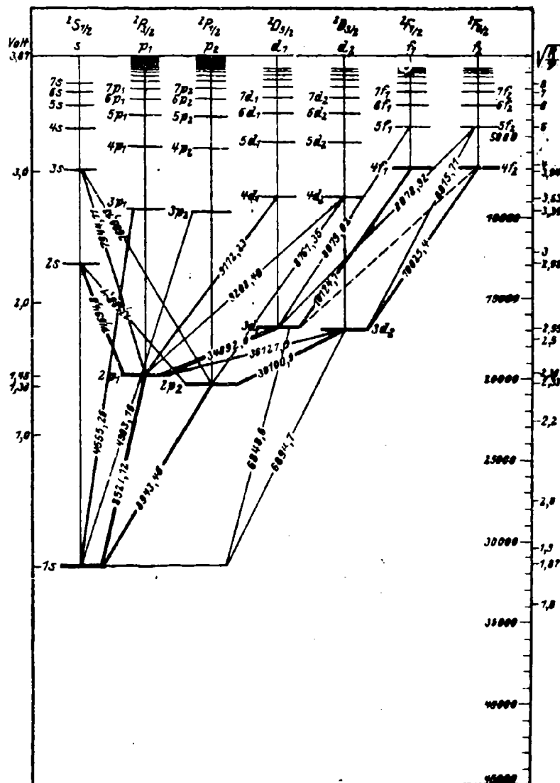
Fig. 84, II, Text S. 60. Niveauschema des Caestum I.
