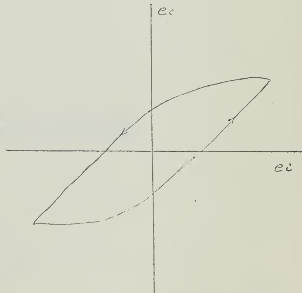
(d) Hysteresis
