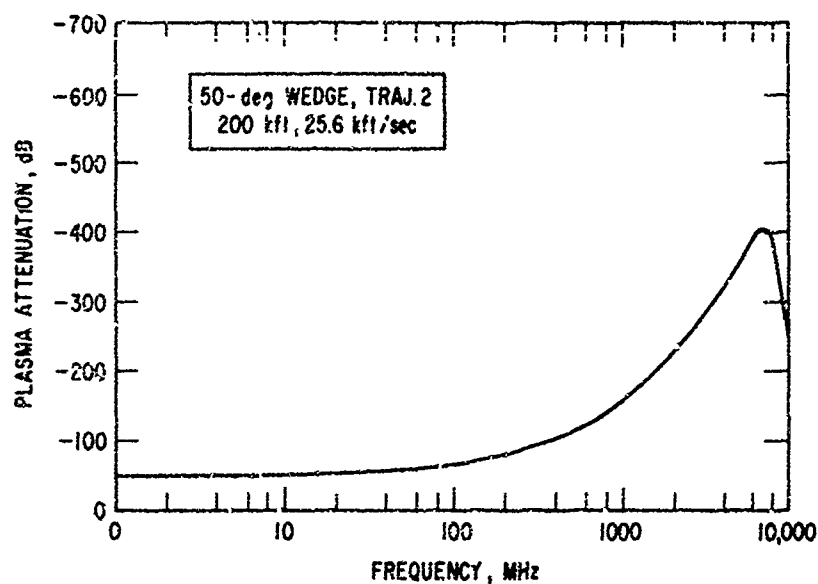
Fig. 44. Plasma Attenuation
