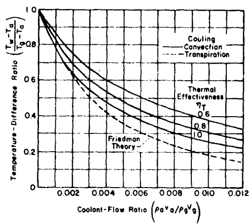
(d) Turbulent flow with radiation Reynolds number = 10^7
