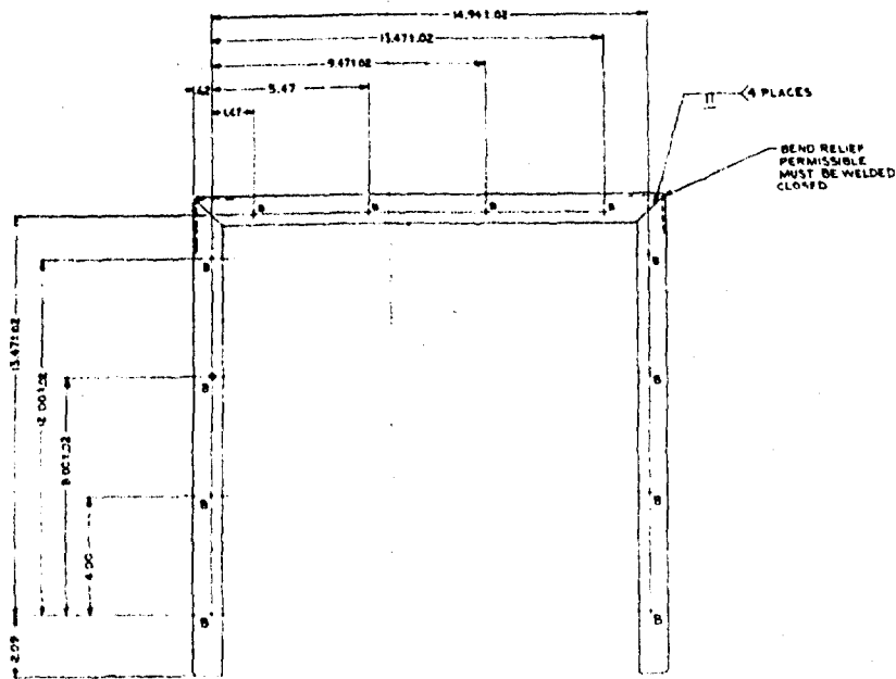
VIEW A-A
