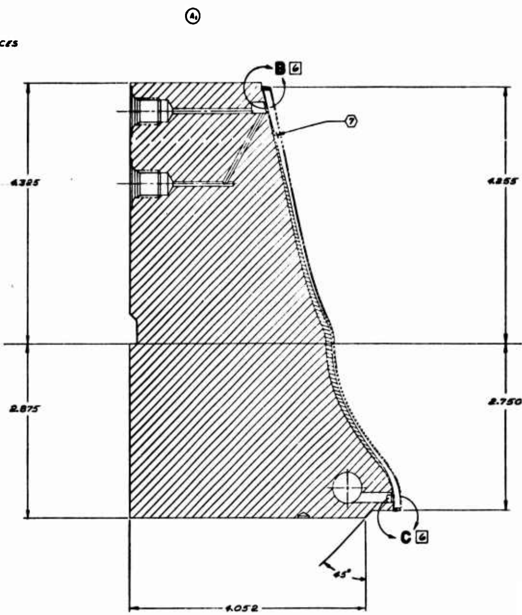
SECTION A-A
