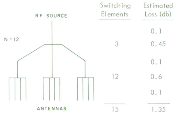
(d) 12-antenna system.
