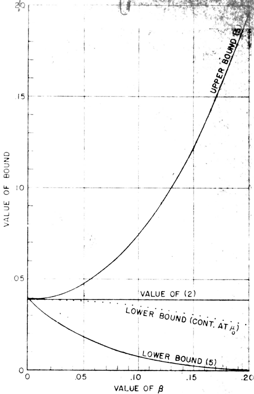
BOUNDS OF (4) FOR n=9, i=8
