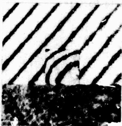
Fig. 6 - Czorchralski Ruby Cube - Twyman-Green Interferogram
