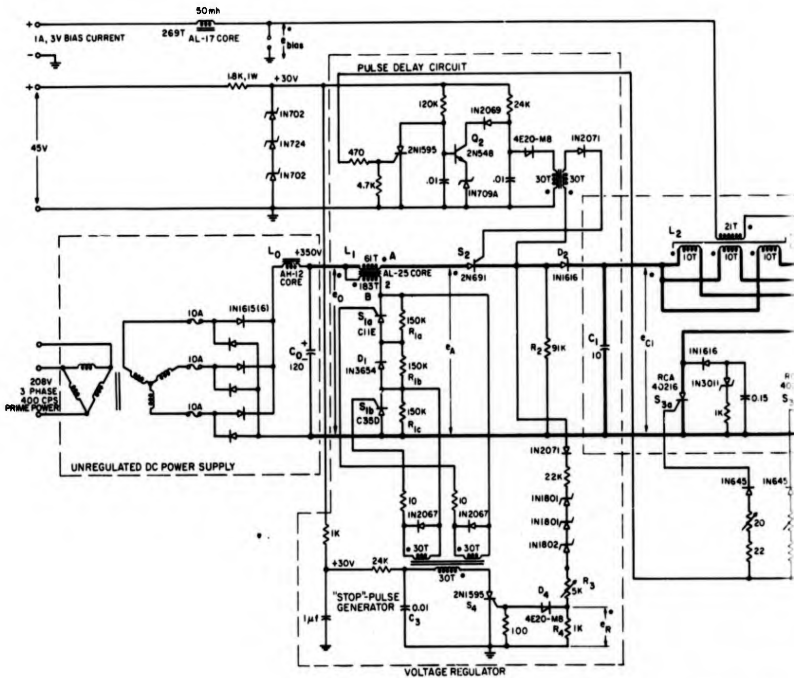
Fig. 5.1 Experimental Pulse Gener
