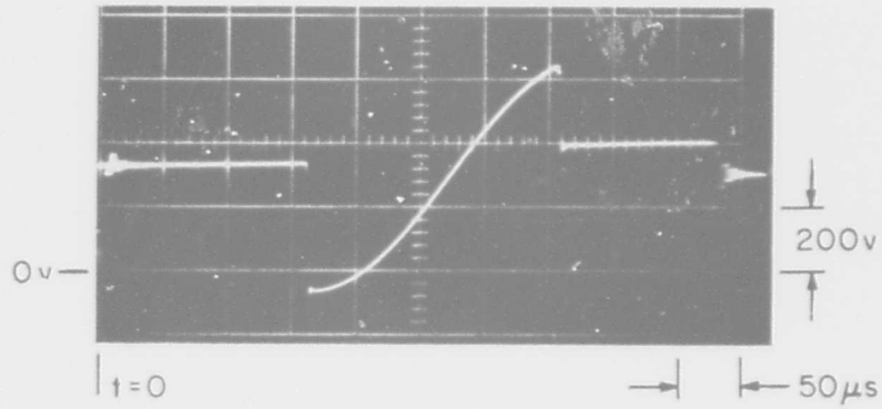
a) Voltage e_A
