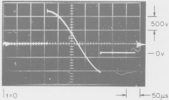
b) Voltage e_B
