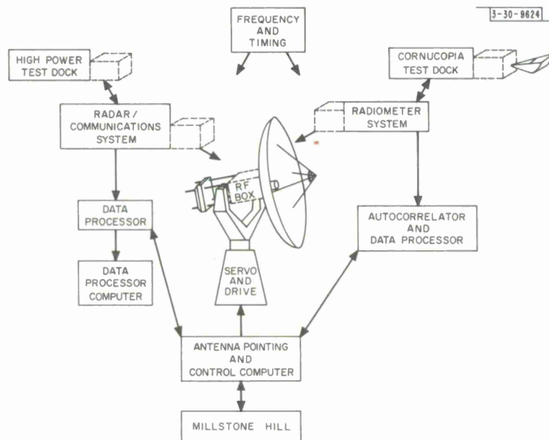
Fig.B-2. Haystack block diagram.
