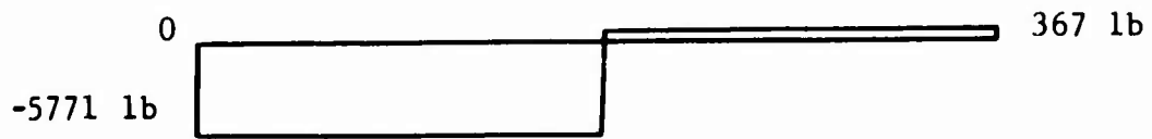
b) Shear Diagram
