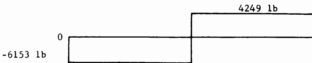
b) Shear Diagram
