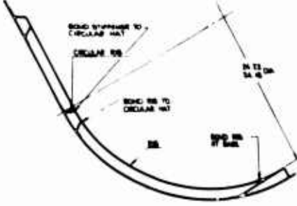
SECTION J-J (ENL. 1/2) SCALE 1/2
