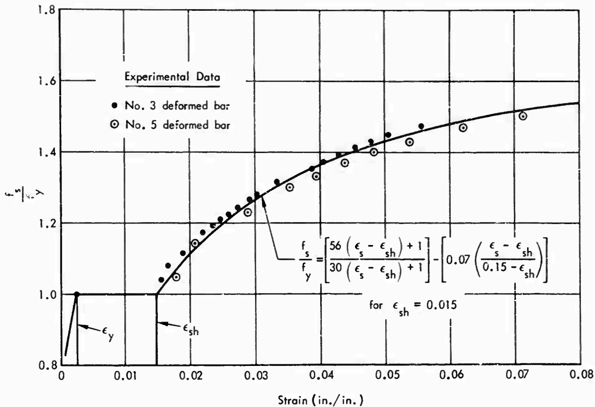
Figure 22. Tensile test data.
