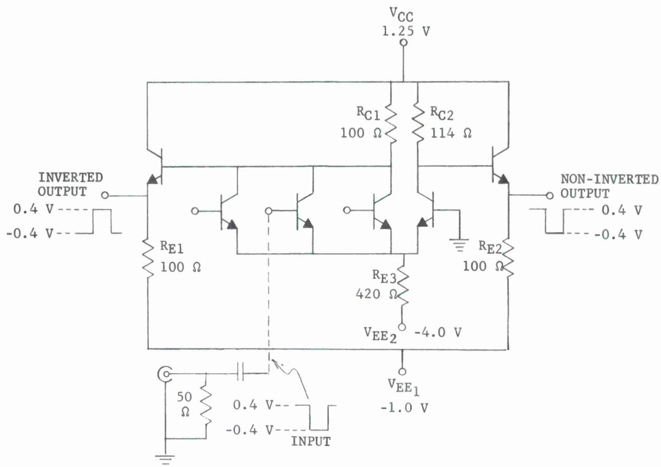
a. Schematic diagram.
