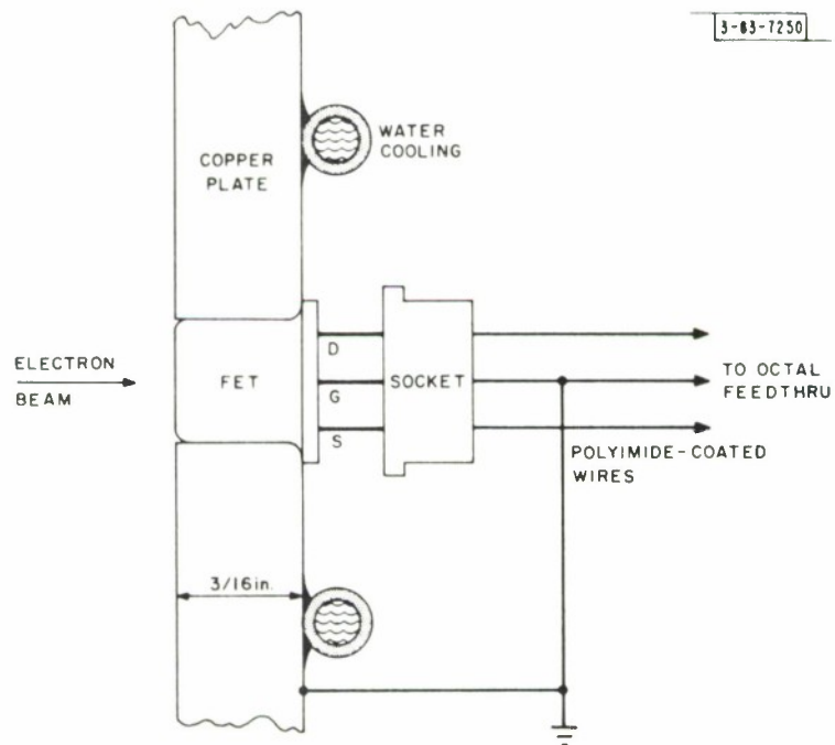
Fig. 2. Transistor mount.
