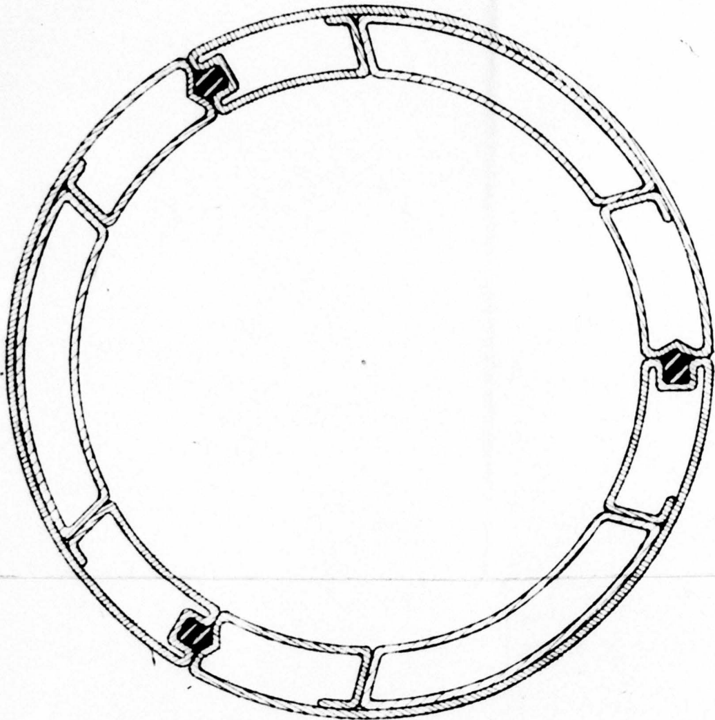
— Section C-C —
