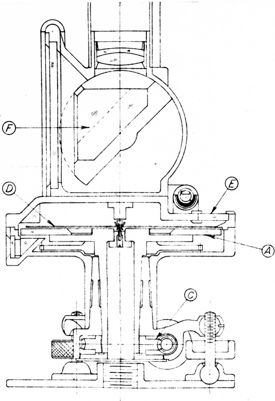
— Section 1-1 —
