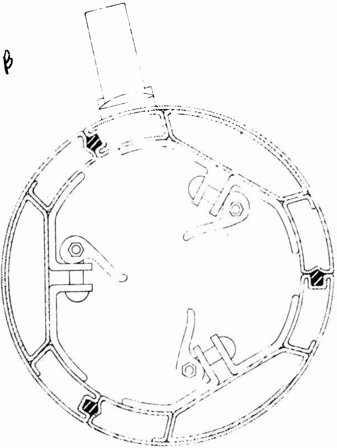
— Section B-B —
