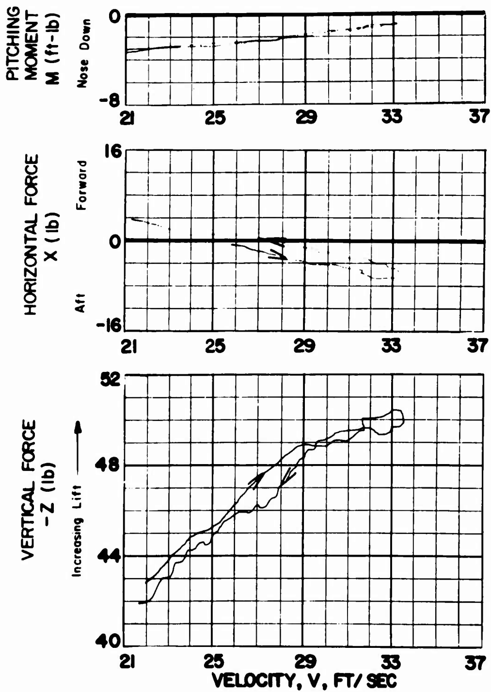
Figure 7p. Static Longitudinal Test Data.
