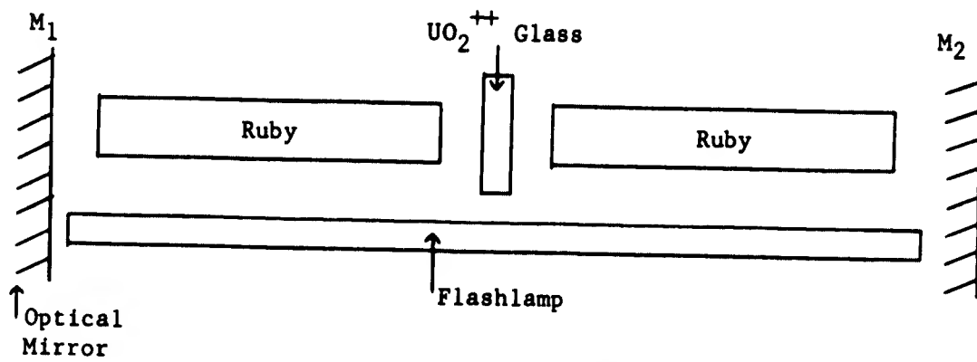
Fig. 10 Laser Apparatus
