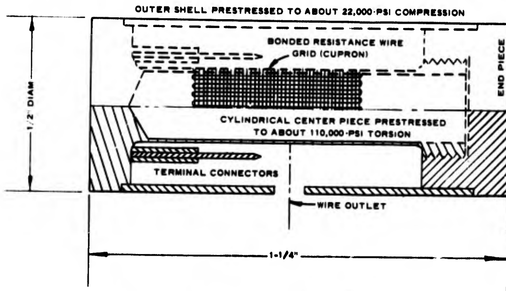
Fig. 15. The Loh or MIT stress meter 1
