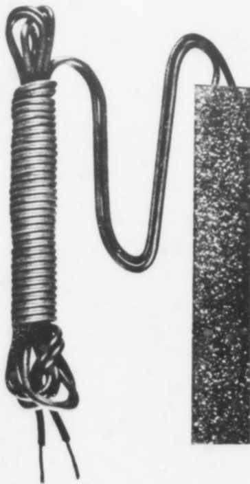
Fig. 9. Polyester mold gage
