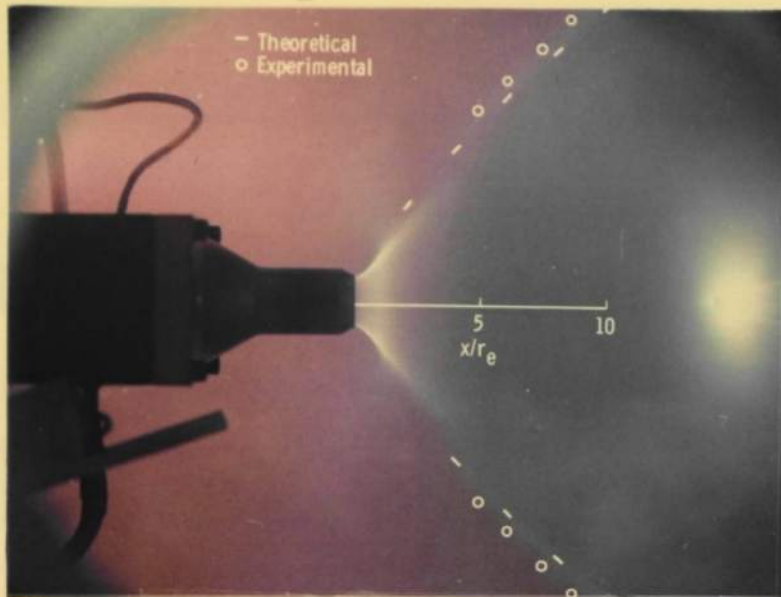
a. \text{CO}_2 , \delta_1 = 60 \text{ deg} , \theta_N = 20 \text{ deg } 36 \text{ min}
