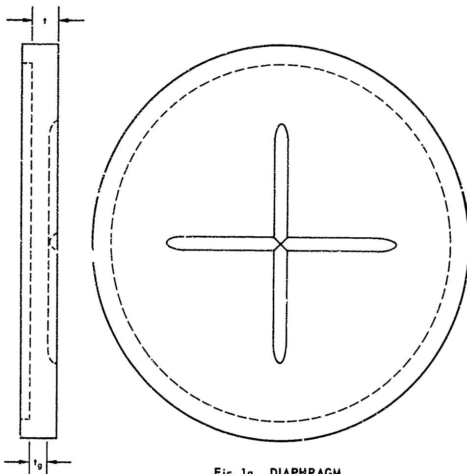
Fig. 1a DIAPHRAGM
