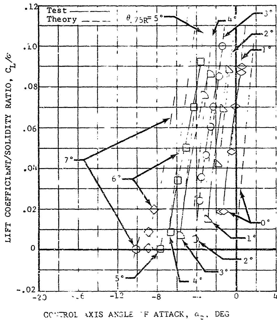
a) C_L/\sigma vs \alpha_c
