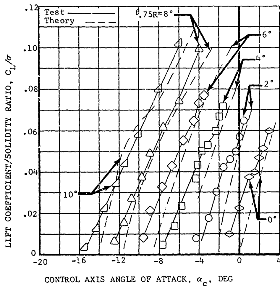
a) C_L/\sigma vs \alpha_c
