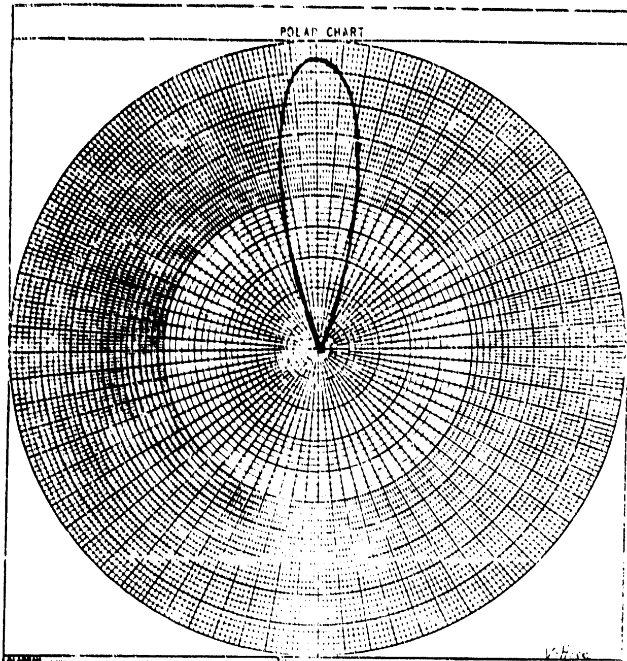
FIGURE 24. 9.0 GHz H-PLANE
