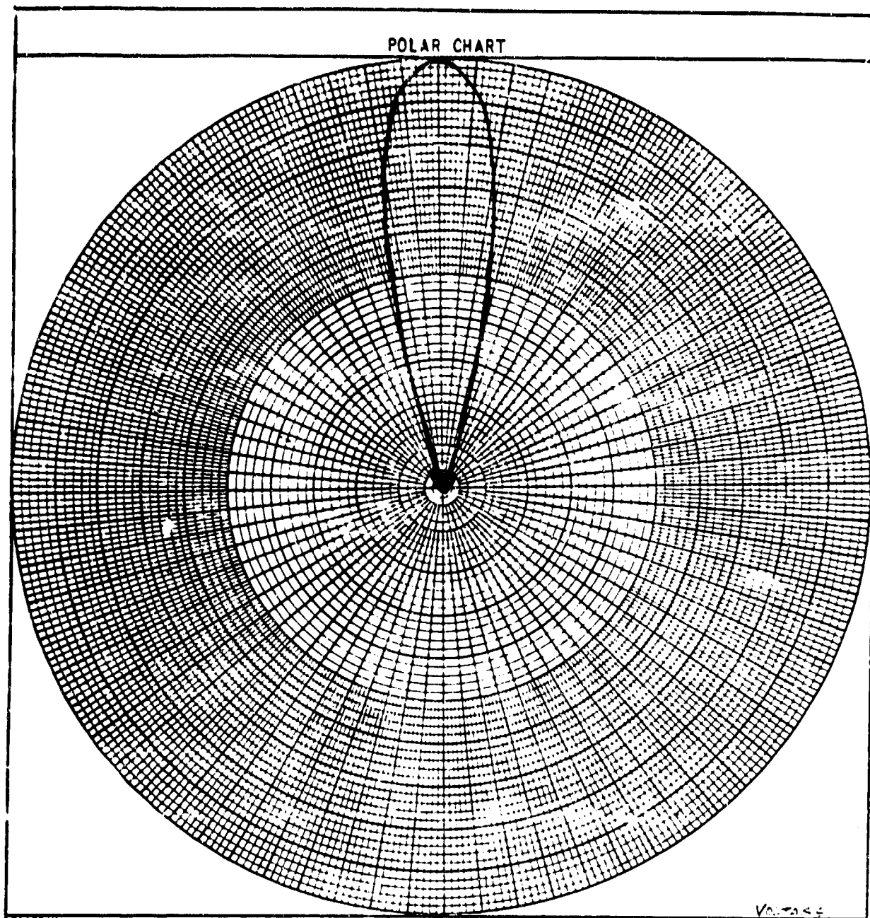
FIGURE 30. 12.0 GHz H-PLANE
