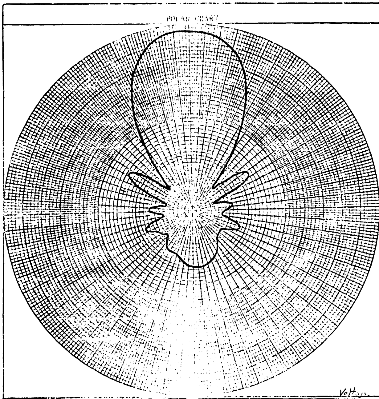
FIGURE 8. 1.5 GHz H-PLANE
