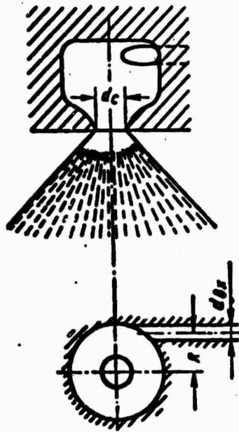
Fig. 28. Swirler.
