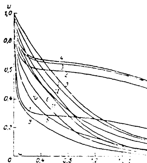
Fig. 1. Solutions of equation (22) — 1—4 and (24) — 5—8, with v_0 = 1.8 ; 9—12 with v_0 = 1 1— t=0.2 ; 2— t=0.4 ; 3— t=0.6 ; 4— t=0.8 5— t=0.2 ; 6— t=0.4 ; 7— t=0.6 ; 8— t=0.8 9— t=0.2 ; 10— t=0.4 ; 11— t=0.6 ; 12— t=0.8
